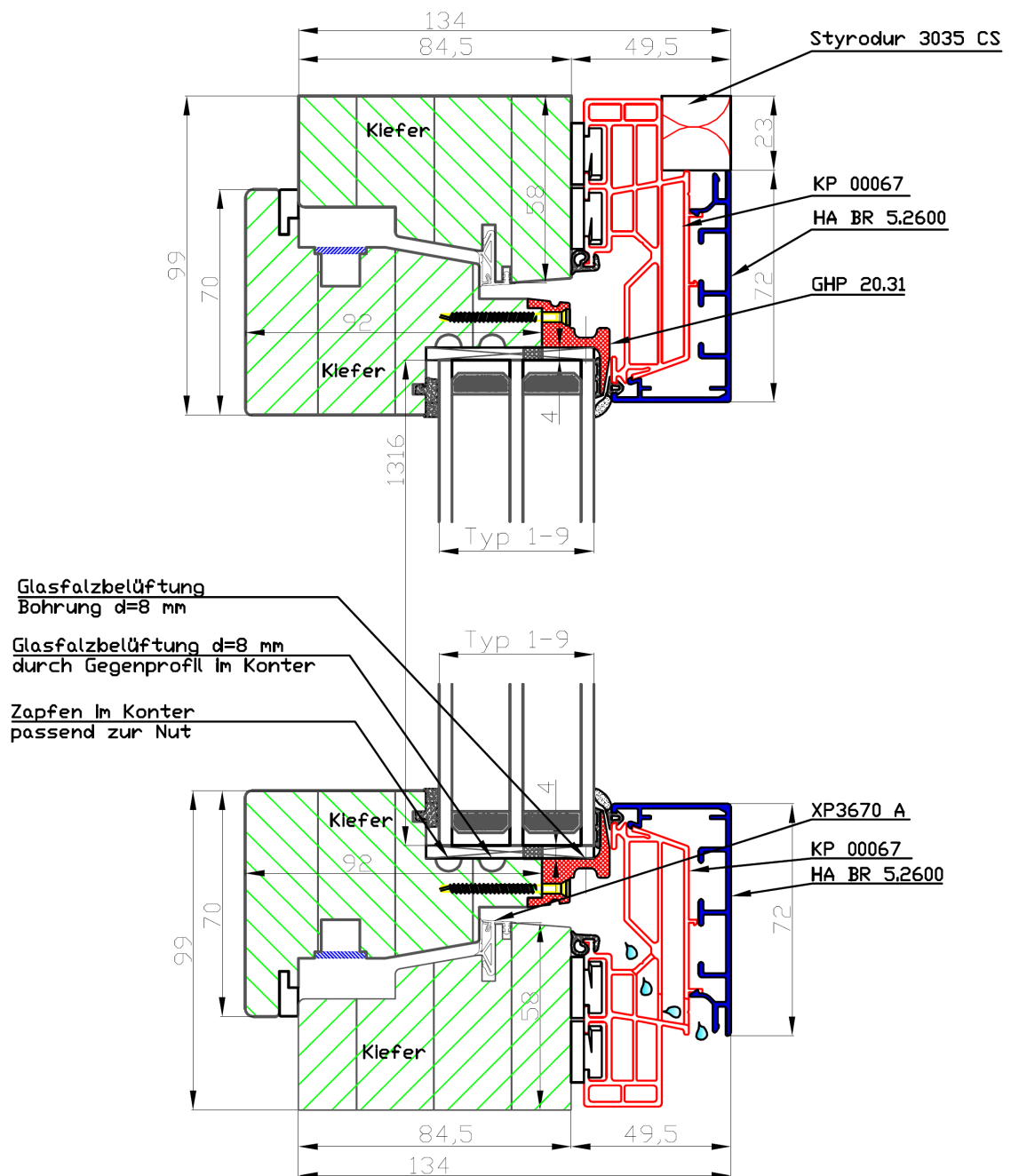
Bild 3 Vertikalschnitt, geprüft wurde mit 8/18/4/18/6 Verglasung (Typ 3)
